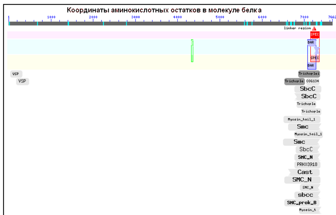
Рис.1. Доменная структура белка XP_002107637.1 Trichoplax adhaerens
