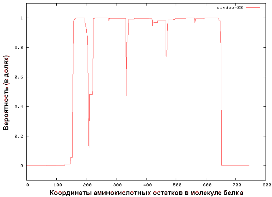
Рис.3. Вероятность формирования альфа-спиральной структуры молекулой белка C(3)G Drosophila melanogaster
