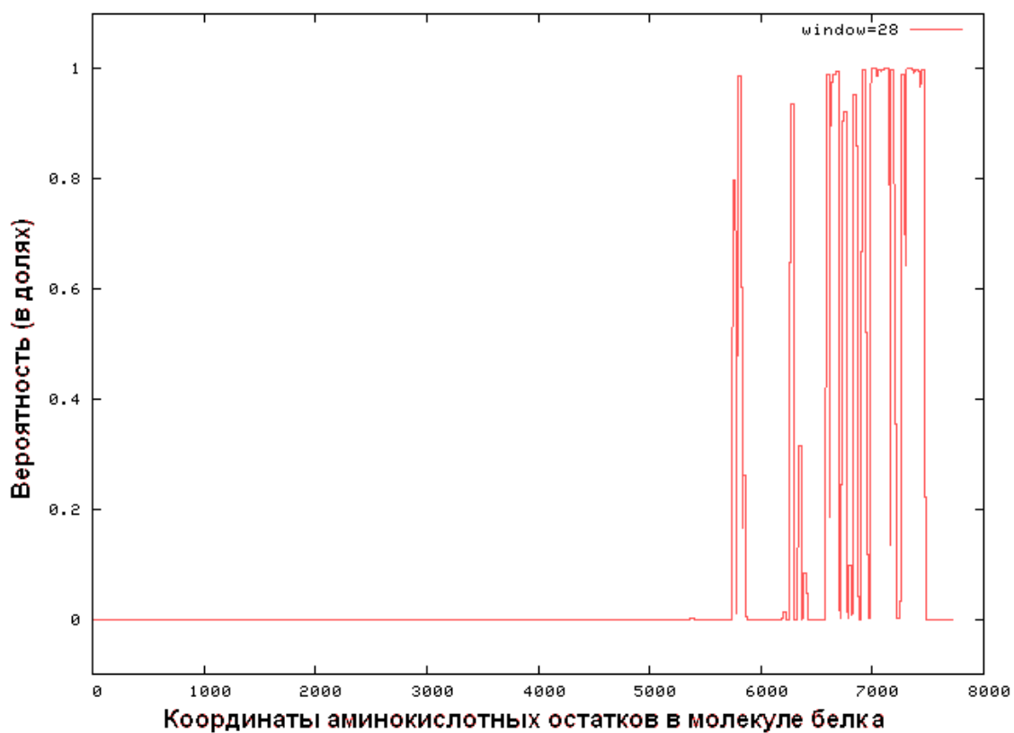
Рис.2. Вероятность формирования альфа-спиральной структуры молекулой белка XP_002107637.1 Trichoplax adhaerens
